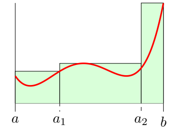
Sur-approximation de l'aire sur la subdivision \mathcal{S} : (a_0, a_1, a_2, a_3)
