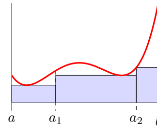
Sous-approximation de l'aire sur la subdivision \mathcal{S} : (a_0, a_1, a_2, a_3)
